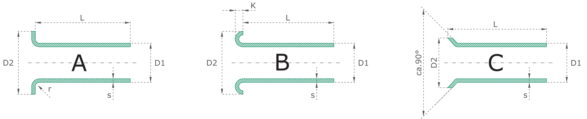
KARTEN A mit Flachkopf KARTEN B mit Rundkopf KARTEN C mit Senkkopf
